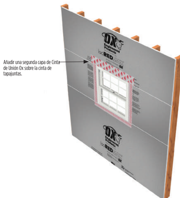
Detalle J - Instalación completada
