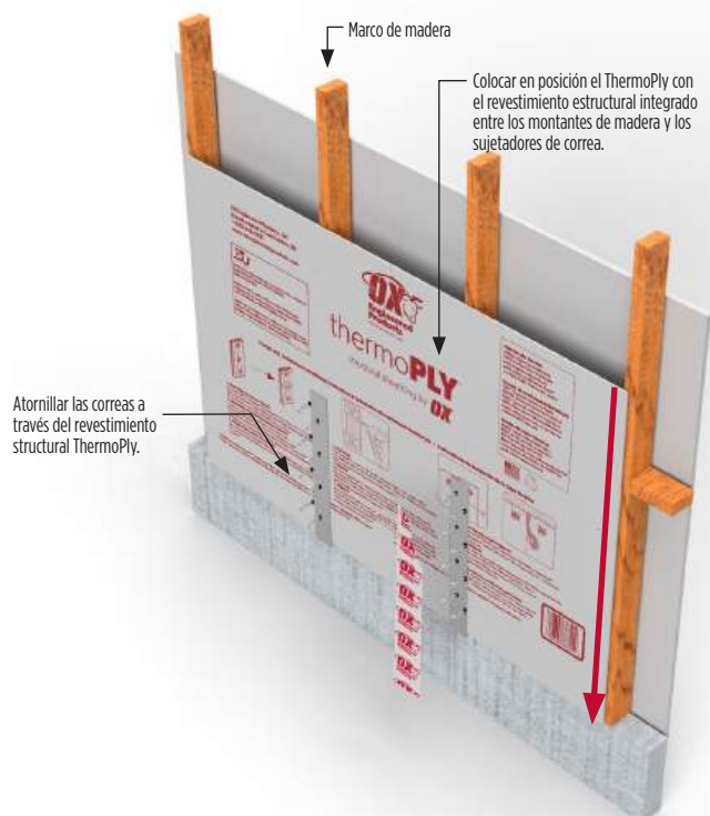
Detalle F
