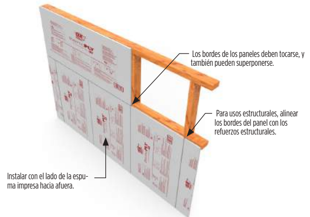
Detalle B
