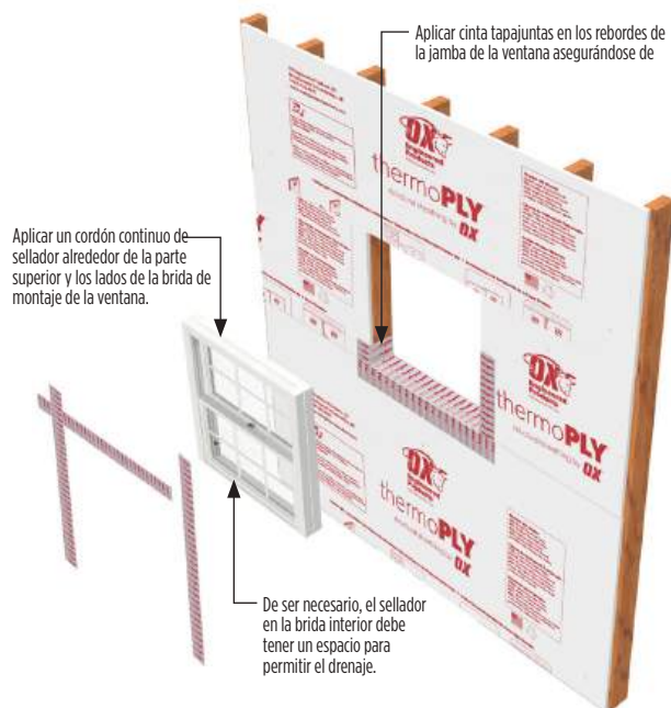
Detalle K-
