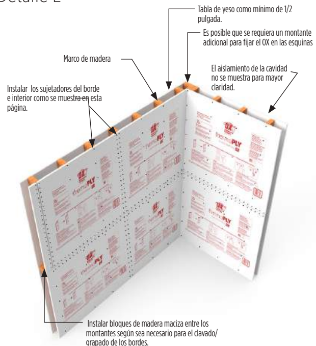
Detalle E
